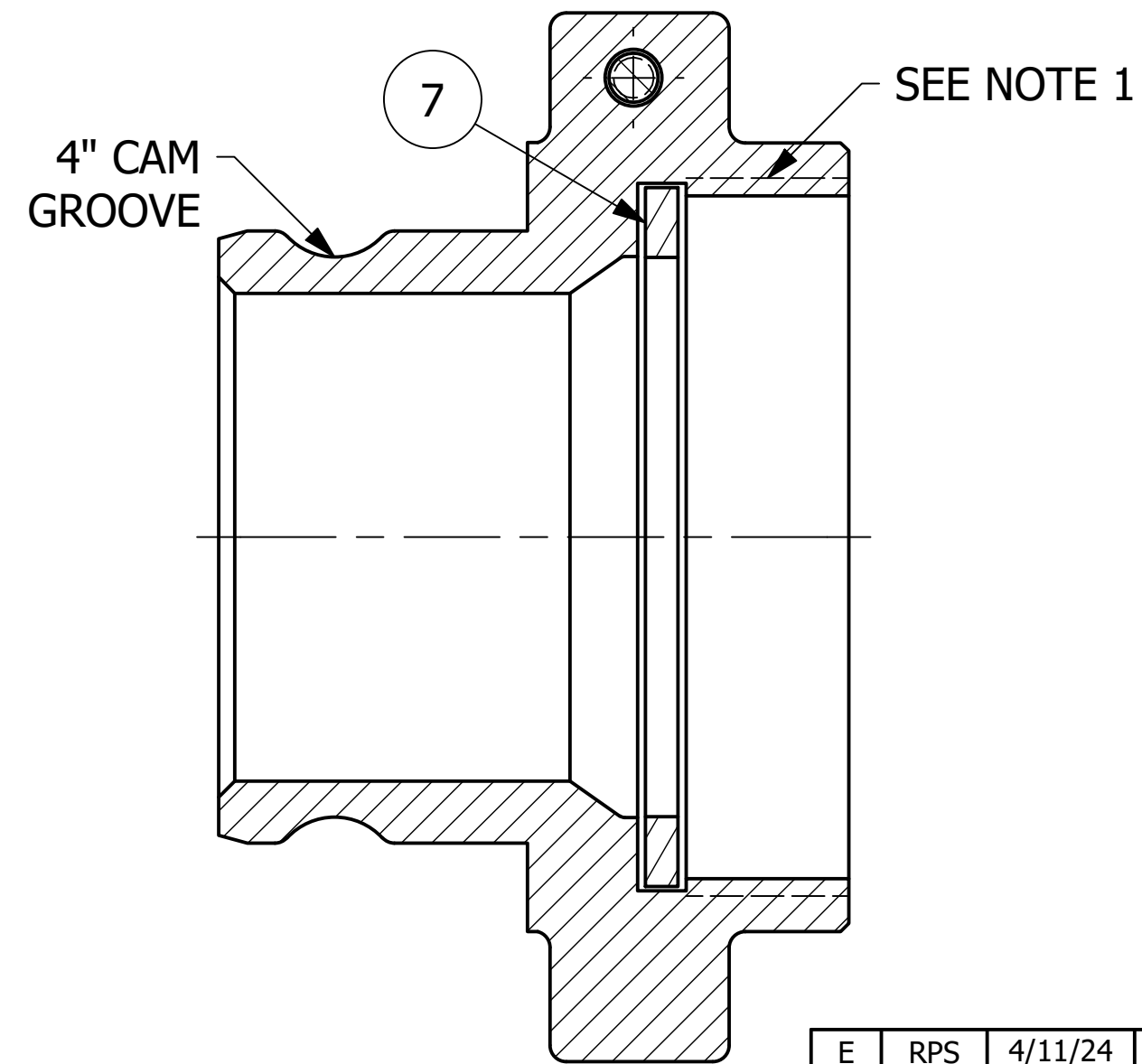
SECTION A-A
