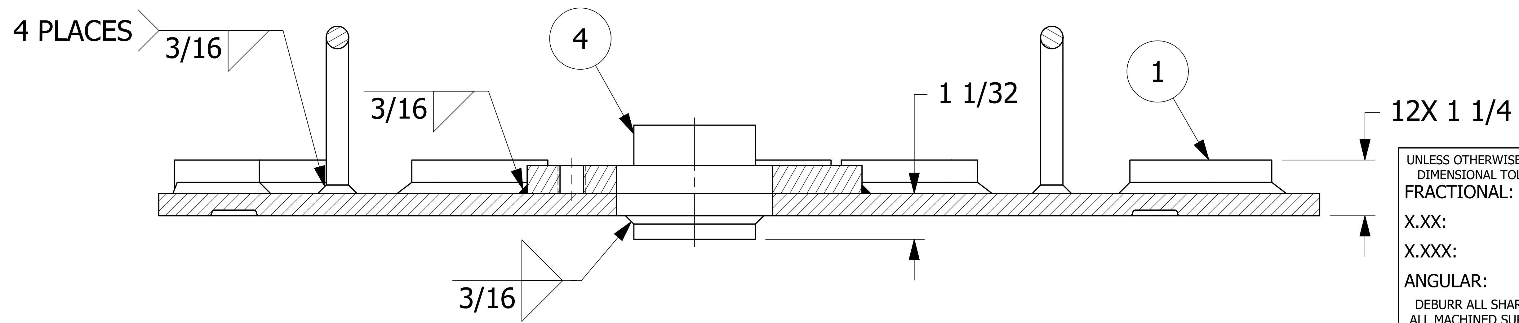
SECTION A-A
