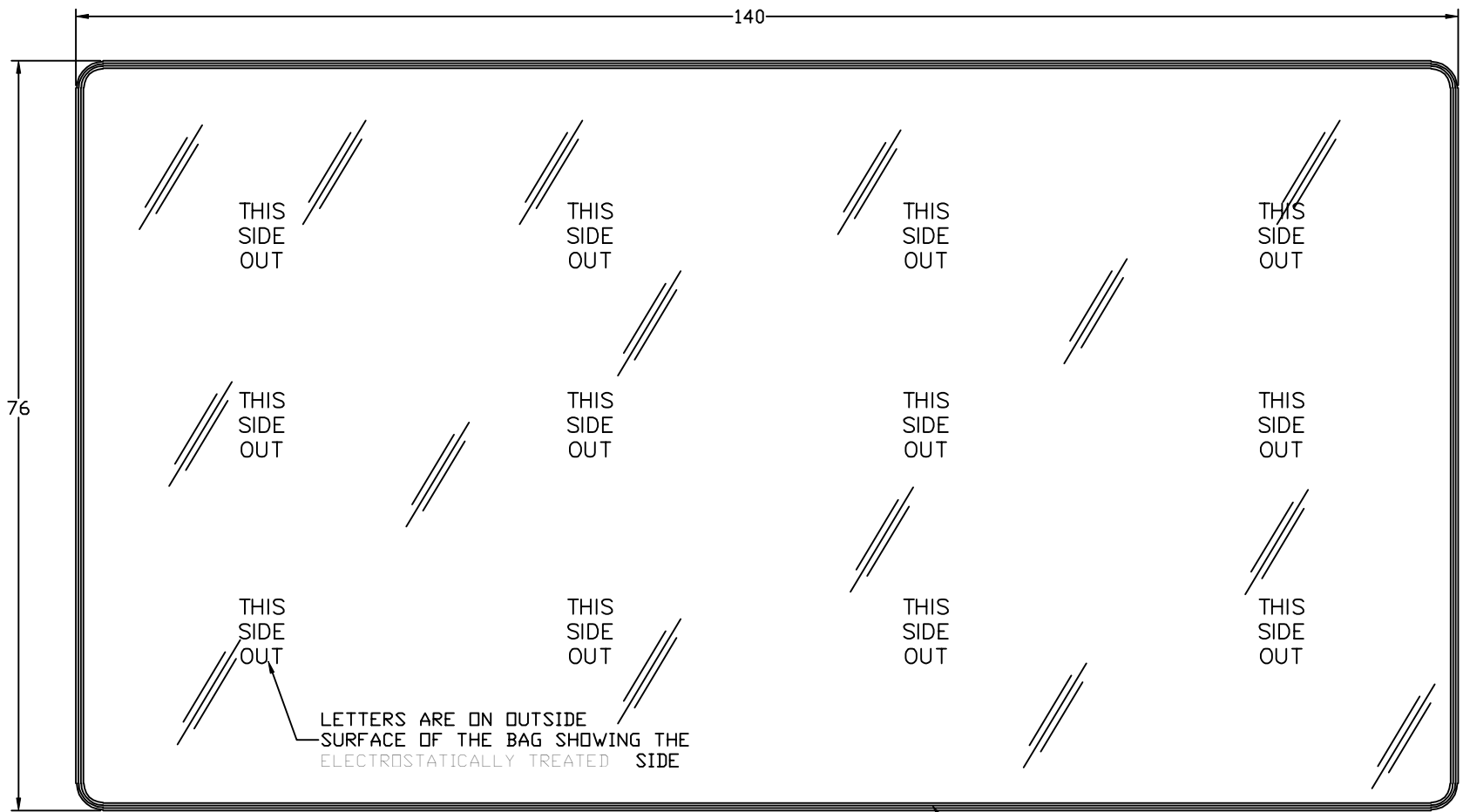
STRECH POSITION 1/4:1 SCALE
